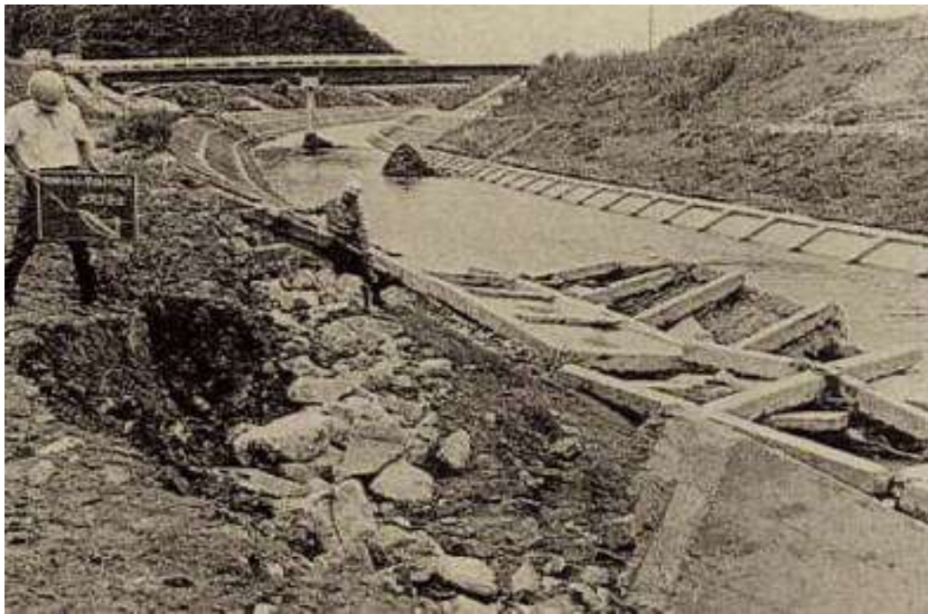
昭和47年7月洪水による白上川の被災状況
